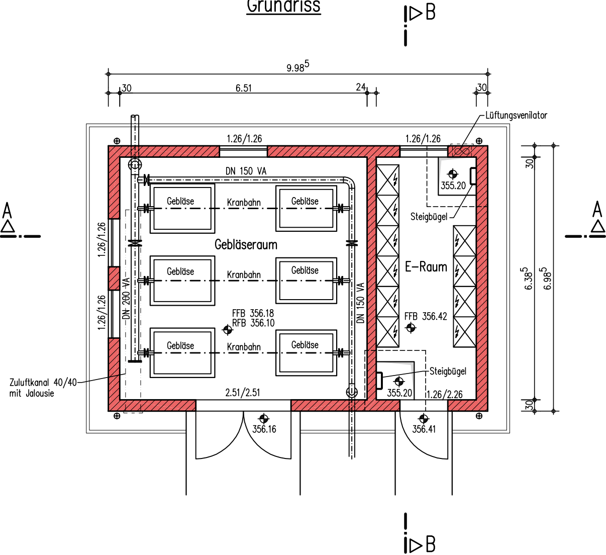
Grundriss
