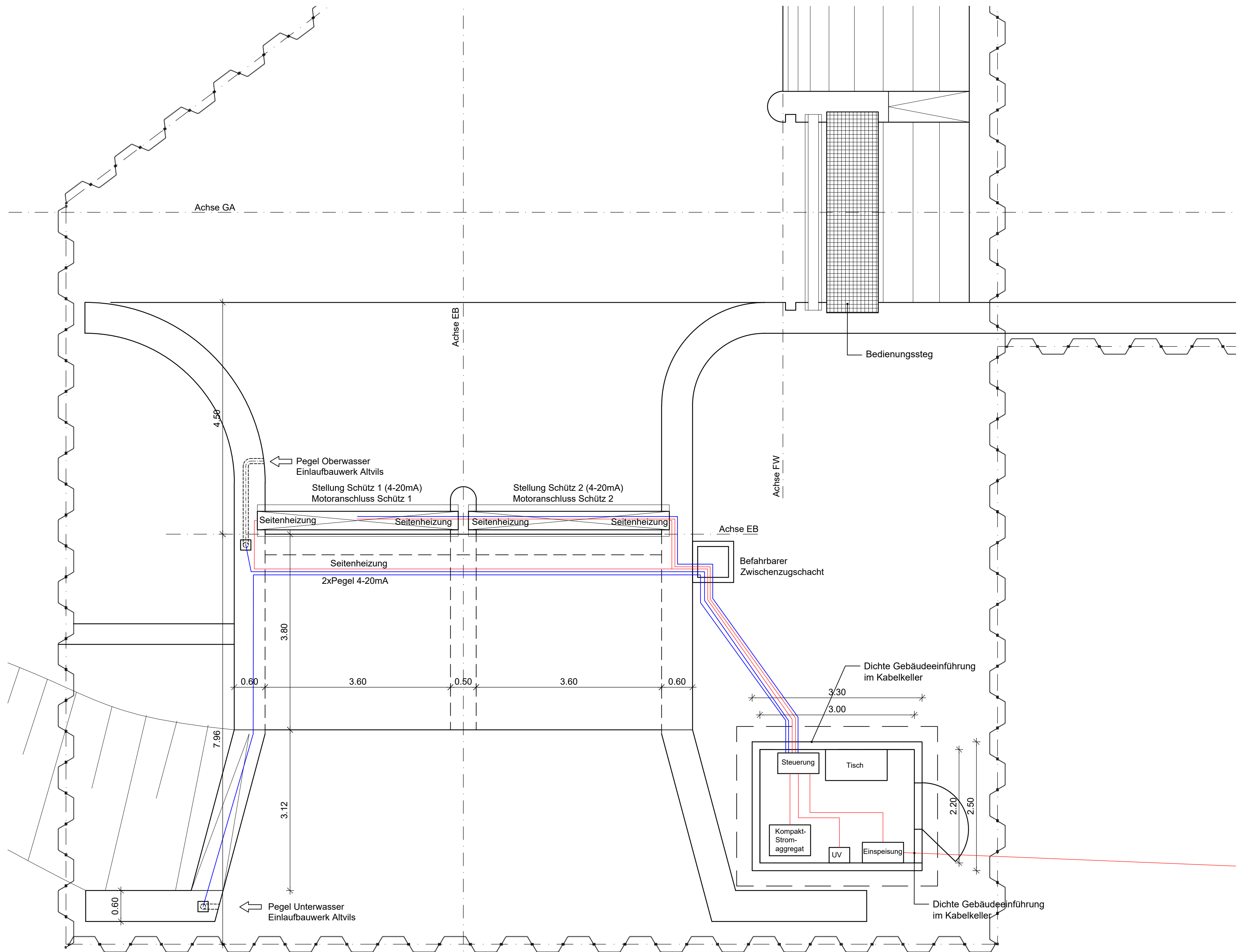
Grundriss Einlaufbauwerk (EB) und Grundablass (GA) M 1:50
