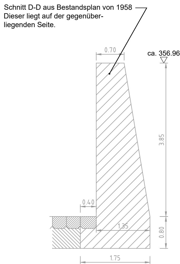
Schnitt I2-I2 (Bestand bleibt unverändert) M 1:50
