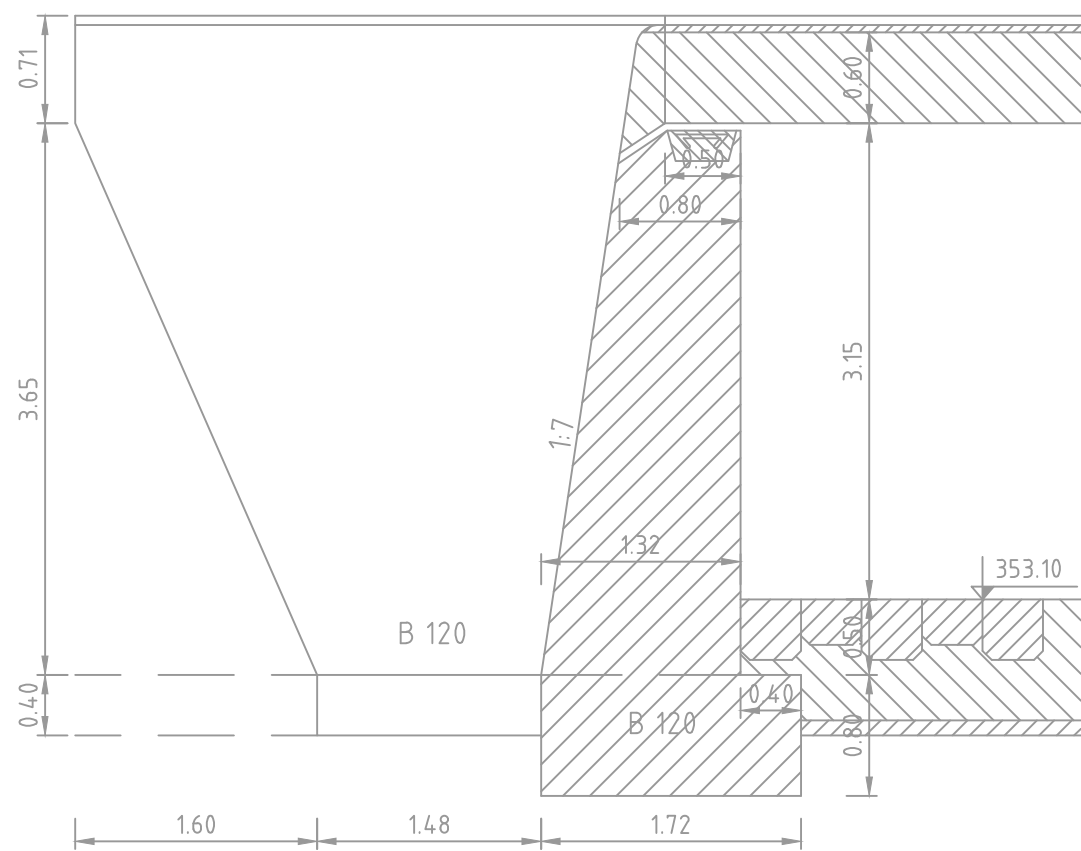
Schnitt J-J (Bestand bleibt unverändert) M 1:50
