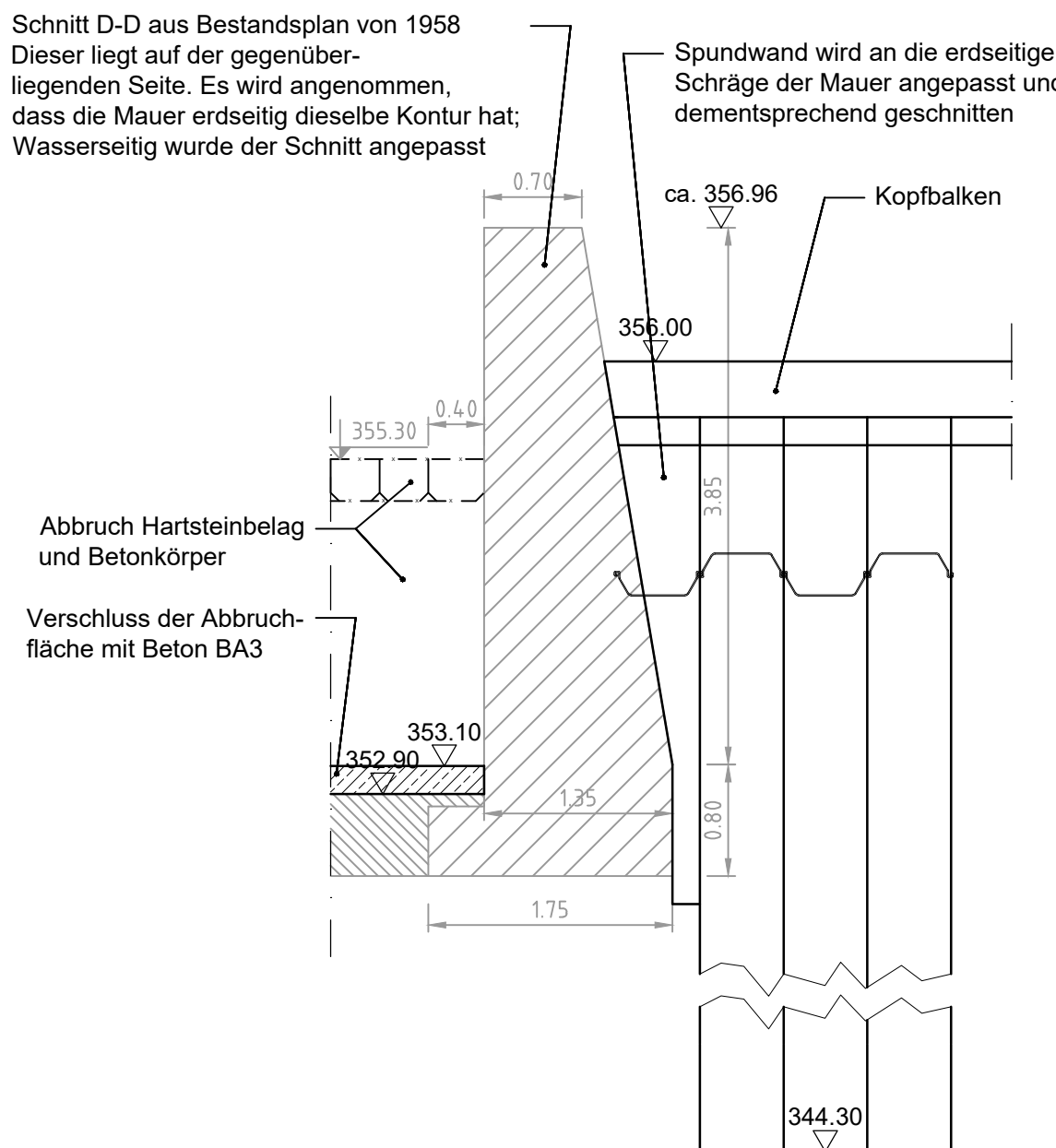
Schnitt I1-I1 M 1:50
