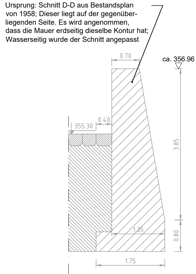
Schnitt I1-I1 (Bestand) M 1:50
