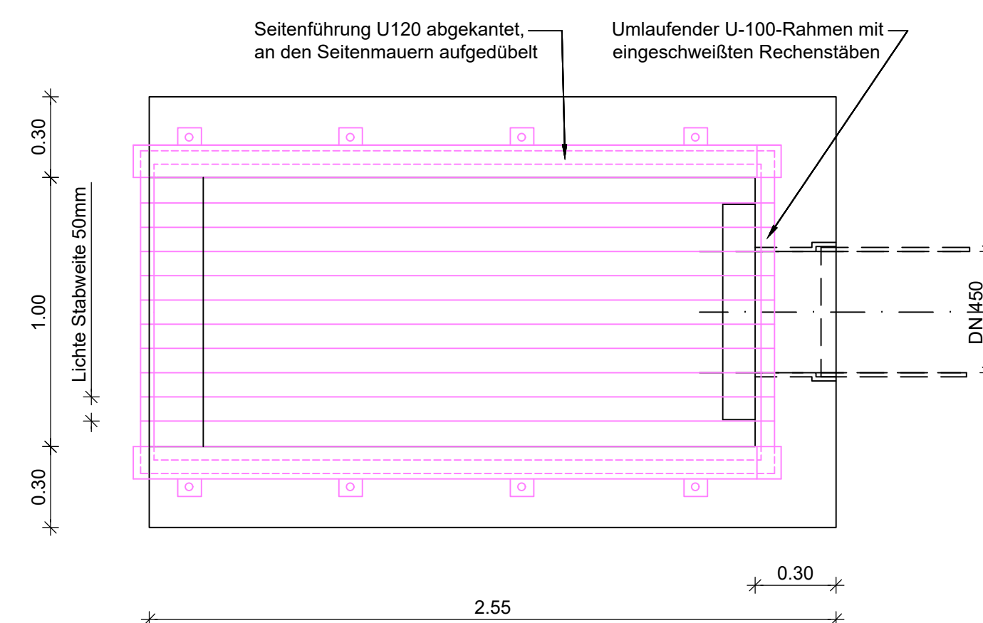
Restwassereinlaufbauwerk (Grundriss) M 1:20
