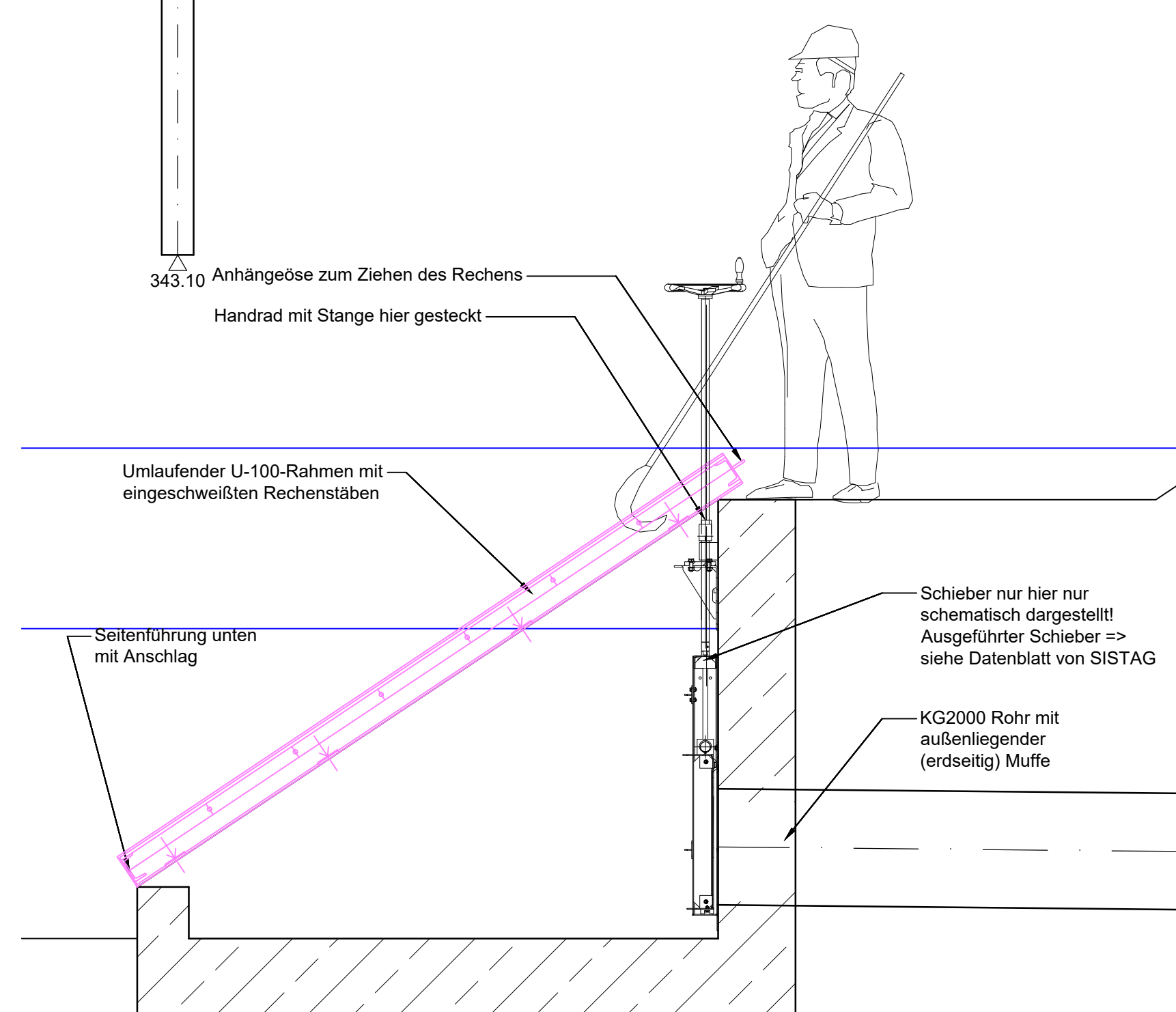
Restwassereinlaufbauwerk (Schnitt K-K) M 1:20
